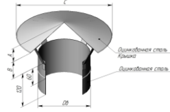
дымоход канал флюгарок ДКУФ
