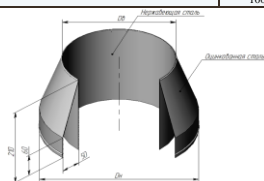
дымоход канал утепленный оголовок ДКУОГ н/о (АISI 430)
