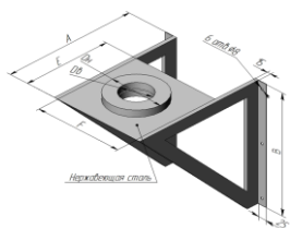
дымоход канал площадка опорная ДУПО нерж
