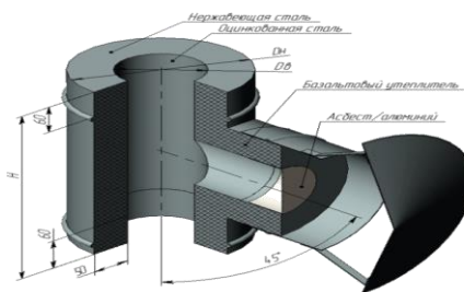
Взрывной клапан
