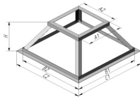
дымоход канал основание секции вертикальной ДКОСВ
