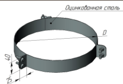
дымоход канал хомут растяжки ДУХР оц
