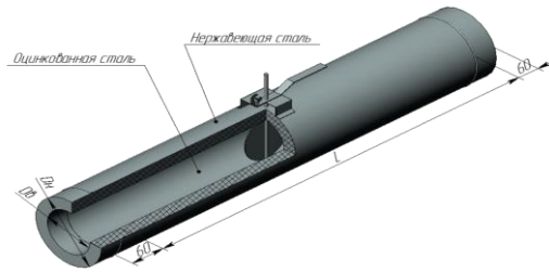
Дроссель клапан утепленный нерж/он
