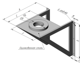
дымоход канал плоская оцинкованная ДКУПО оц
