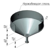
дымоход канал заглушка конденсатосборник ДКЗС (AISI 430)
