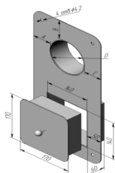
дымоход канал панель ДКП н/о
