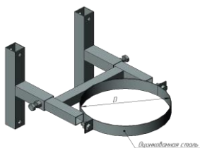
дымоход канал кронштейн секции вертикальной ДУКСВ
