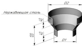
дымоход канал адаптер переход ДУАП нерж (AISI 321)
