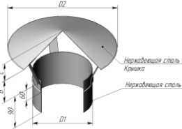
дымоход канал флюгарок ДКУФ (AISI 430)
