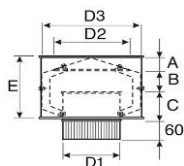
дымоход канал дефлектор ДКД (AISI 430)
