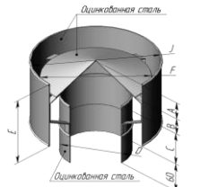
дымоход канал дефлектор ДКД он
