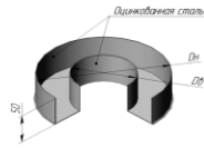
дымоход канал утепленный стакан ДКУС о/о
