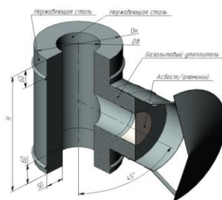
Вращающийся клапан нерж/нерж
